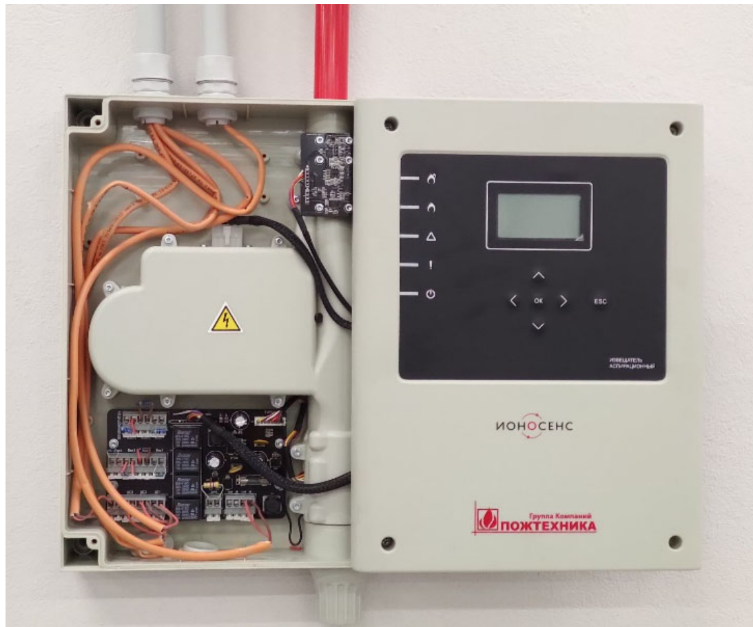
Рисунок 13 – Крепление крышки при монтаже извещателя
