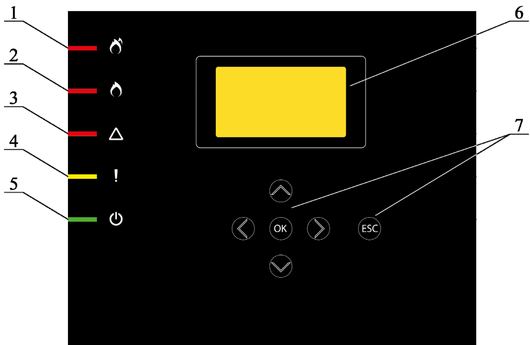
Рисунок 4 – Органы управления и индикации извещателей ИП 233-3, ИП 233-4, ИП 233-5, ИП 233-6
