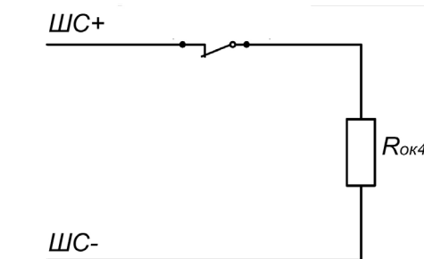
Рисунок 7 – Схема подключения реле «Неисправность»
