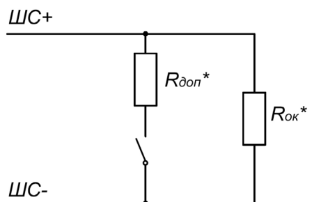
Рисунок 6 – Схема подключения реле «Внимание», «Пожар 1», «Пожар 2»
