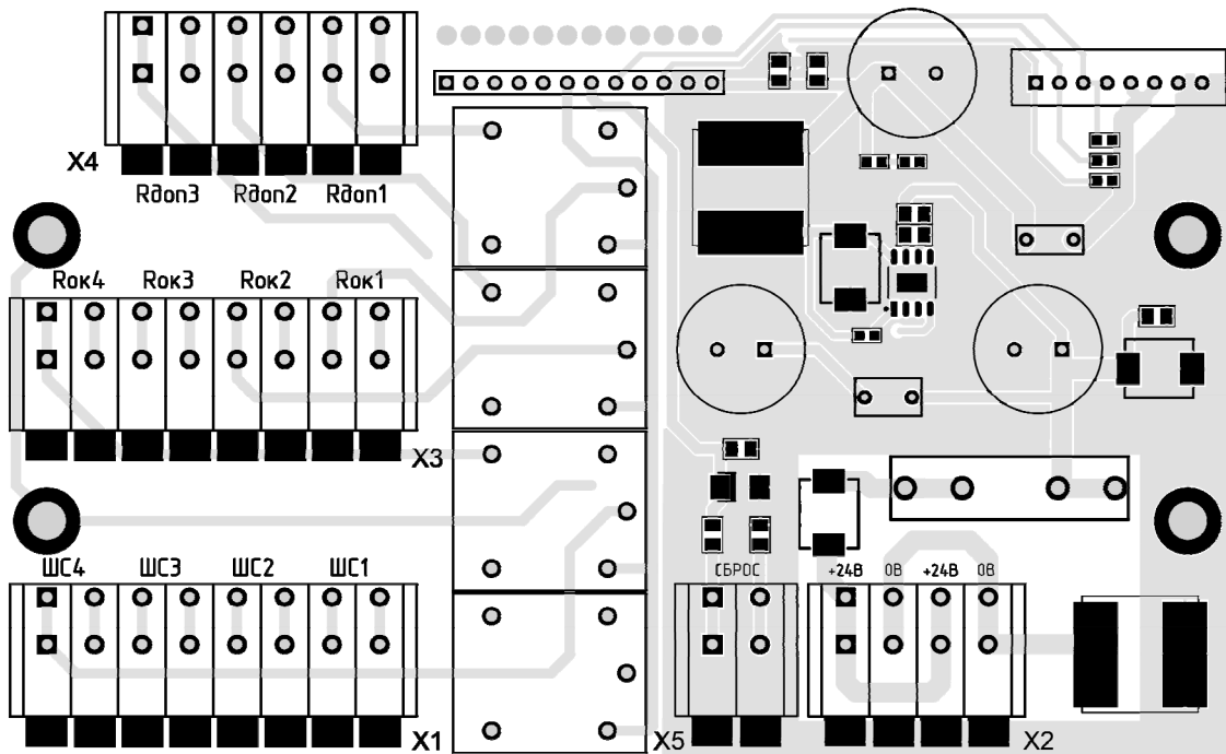
Рисунок 9 – Расположение терминалов на коммуникационной плате
