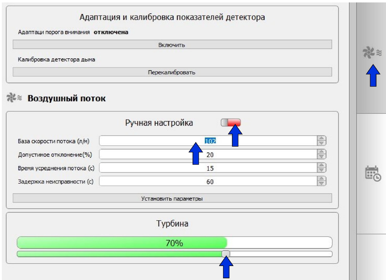
Рисунок 15 – Установка скорости турбины
