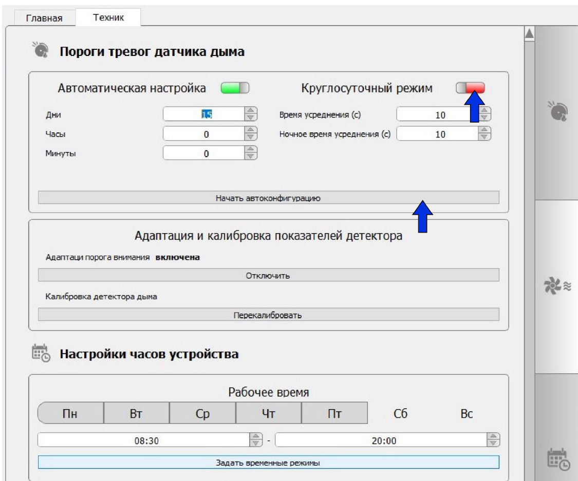
Рисунок 20 – Автоматическое конфигурирование порогов тревог «день/ночь»
